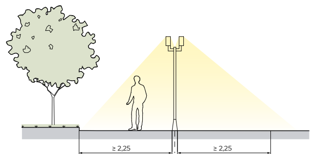
ИЛЛ. 3.6. ОСЕВАЯ СХЕМА РАСПОЛОЖЕНИЯ ОПОР ОСВЕЩЕНИЯ
