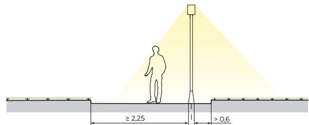
ИЛЛ. 3.5. ОДНОСТОРОННЯЯ СХЕМА РАСПОЛОЖЕНИЯ ОПОР ОСВЕЩЕНИЯ
