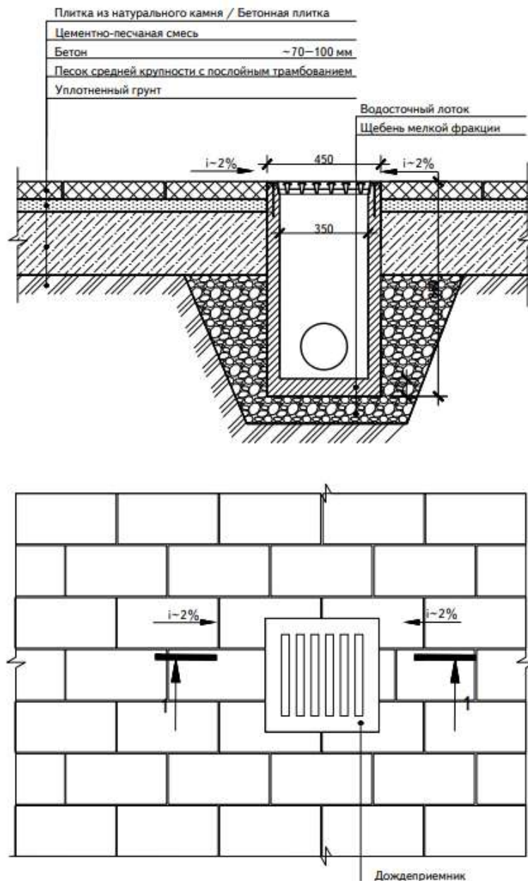
Илл. 1.2.14. ПРИНЦИПИАЛЬНАЯ СХЕМА УСТРОЙСТВА ДОЖДЕПРИЕМНИКА НА ТРОТУАРЕ
