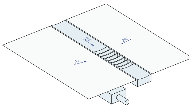
ЛИНЕЙНЫЙ ВОДООТВОД
